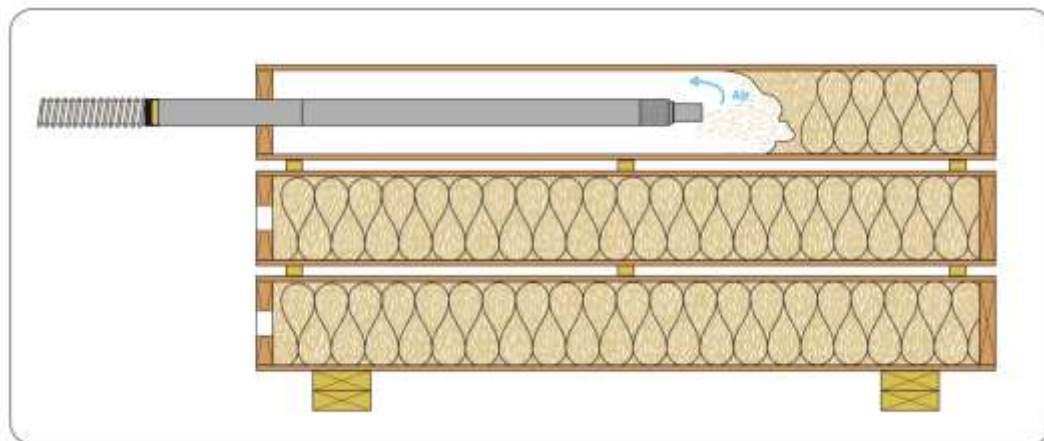
Figure 6: Principe d'insufflation par lisse basse
